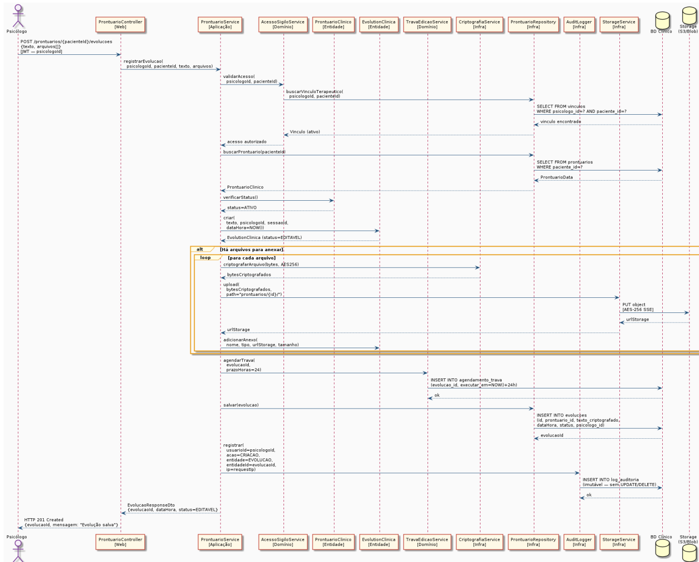
Figura: C4 — Sequência: ProntuarioService.registrarEvolucao()
