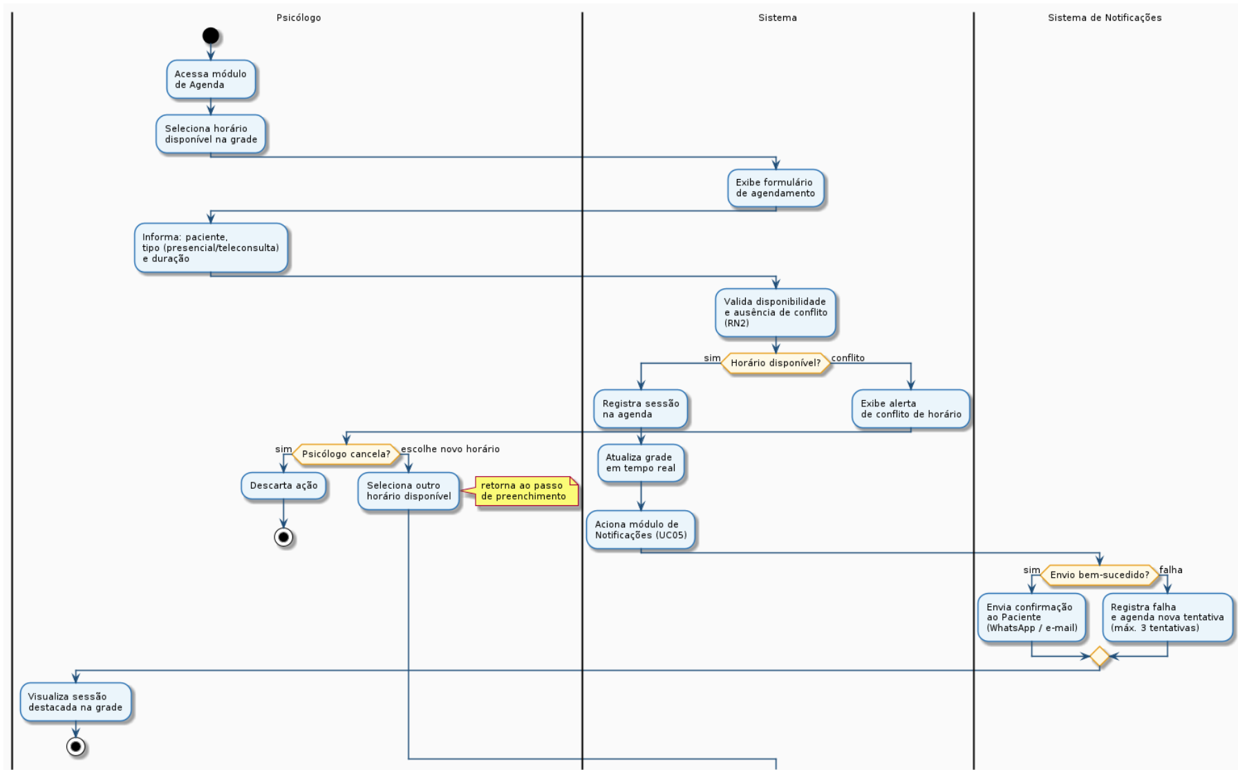
Figura: C1 — BPMN: Processo de Agendamento de Sessão
