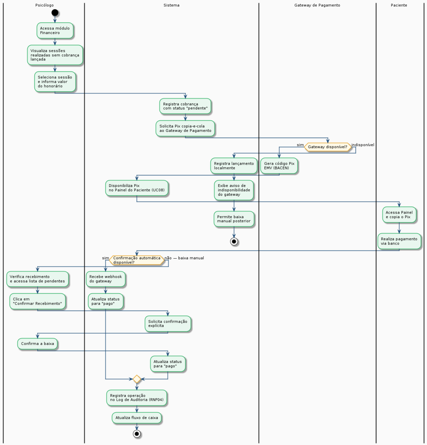
Figura: C1 — BPMN: Processo de Gestão de Cobrança e Pagamento
