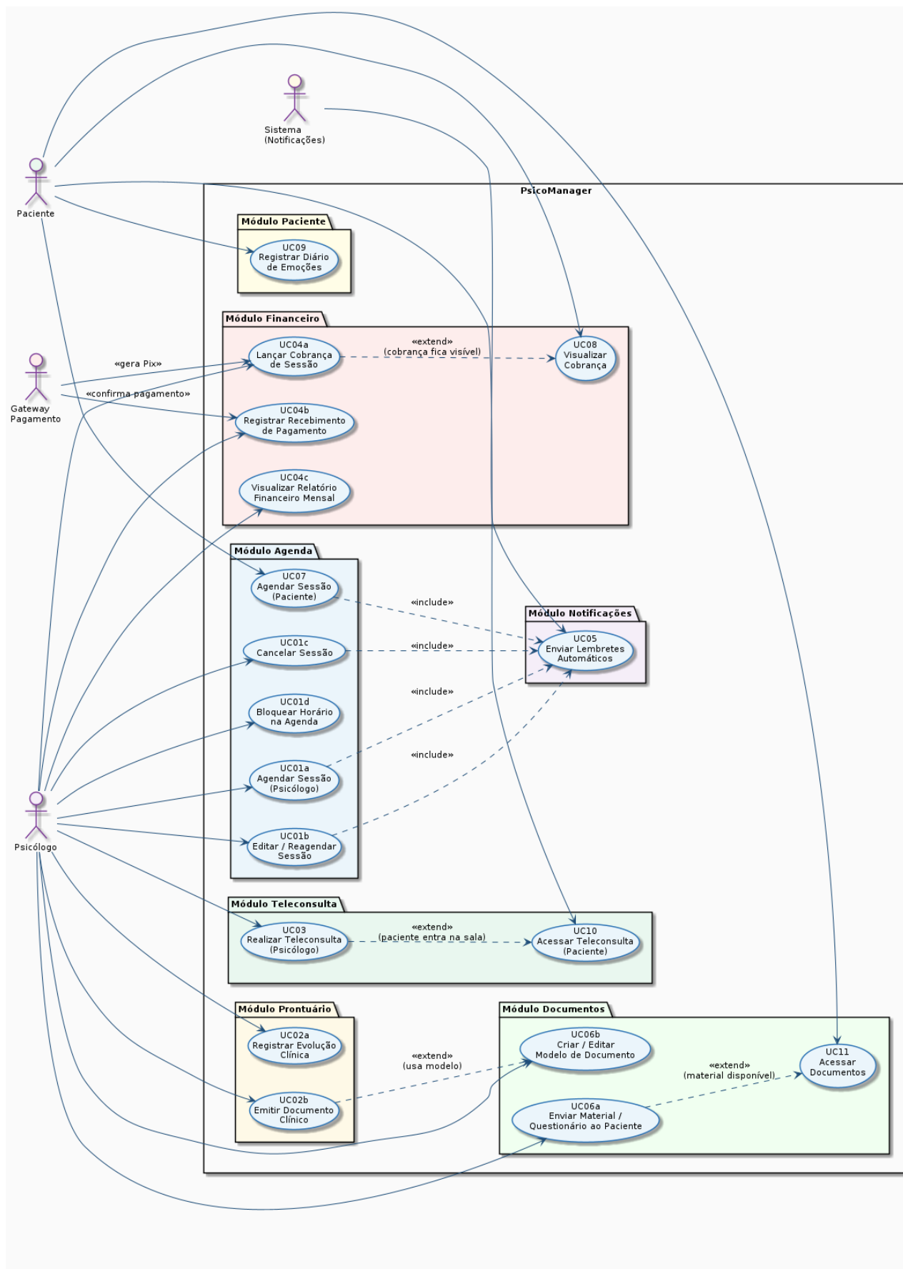
Figura: C1 — Diagrama de Casos de Uso
