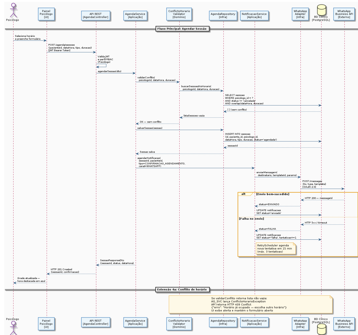
Figura: C3 — Diagrama de Sequência entre Componentes (UC01a)
