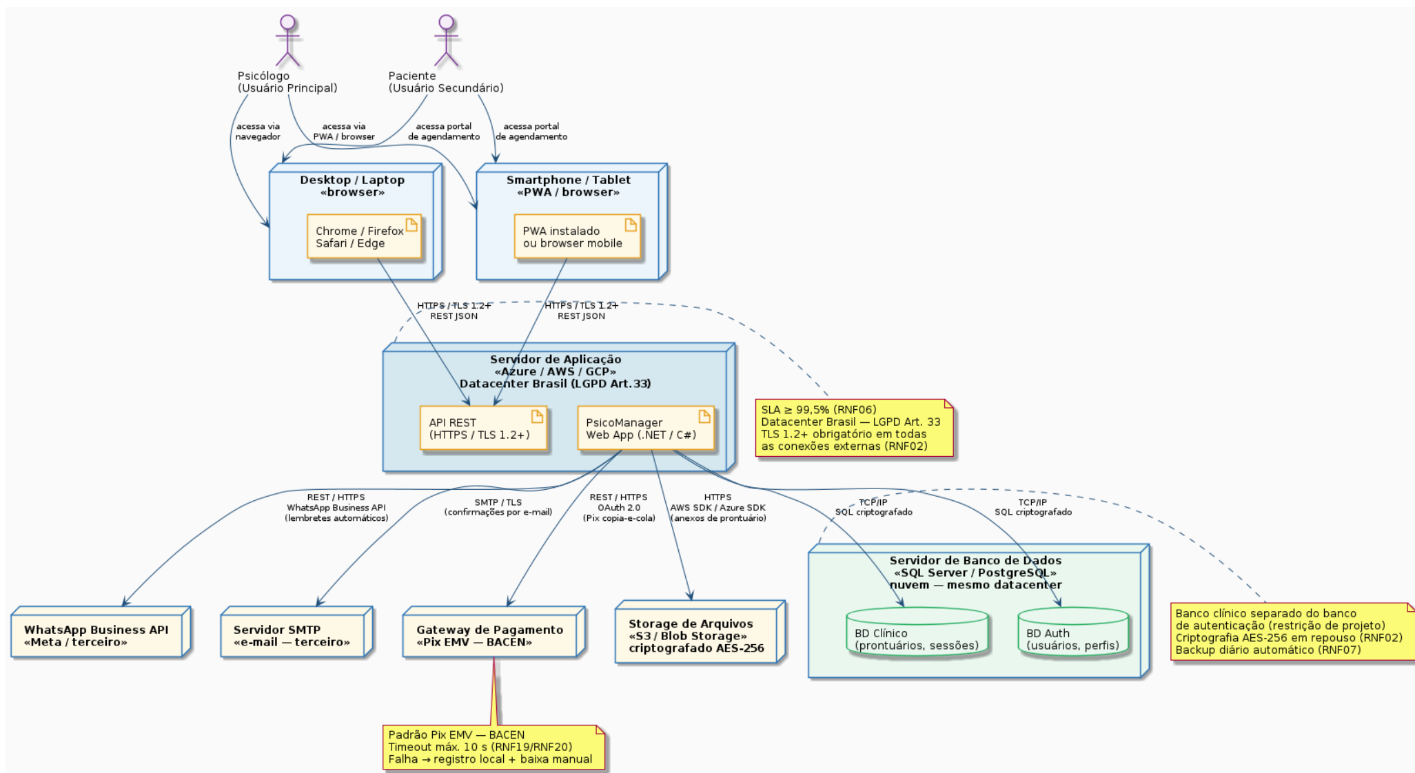
Figura: C1 — Diagrama de Implantação
