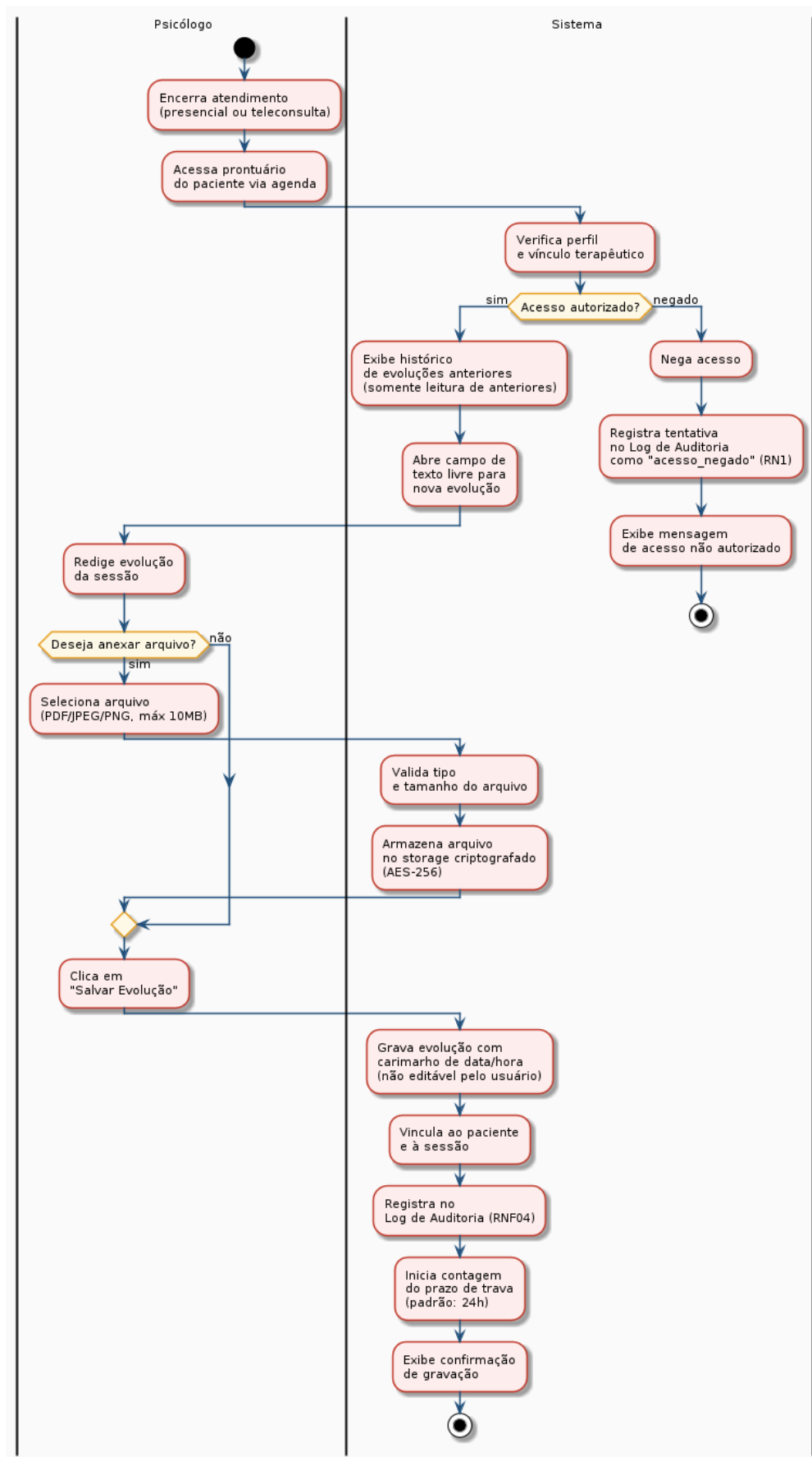
Figura: C1 — BPMN: Processo de Registro de Prontuário Clínico
